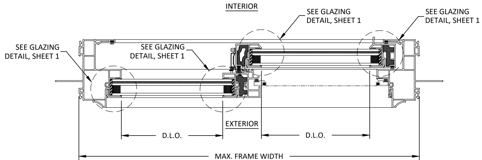
C 4 HORIZONTAL SECTION NAIL FIN
