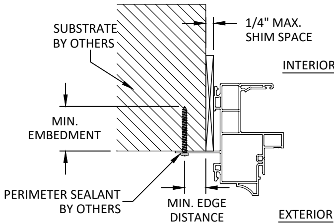
D 5 ANCHOR DETAIL NAIL FIN (JAMB)
